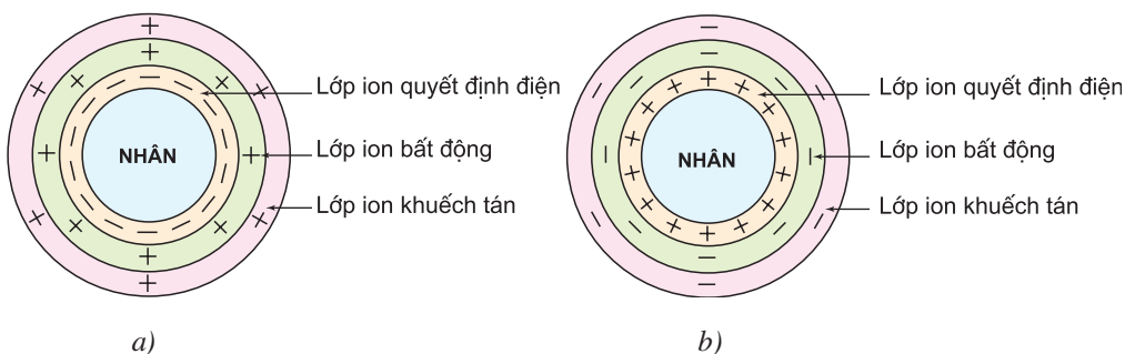
Hình 7. Sơ đồ cấu tạo của keo đất a) Keo âm ; b) Keo dương
